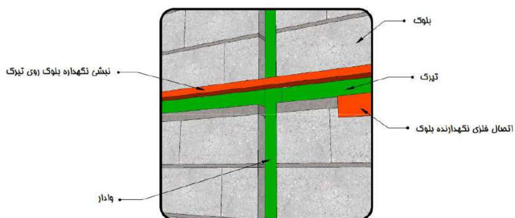
جزئیات اتصال تیرک به وادر
