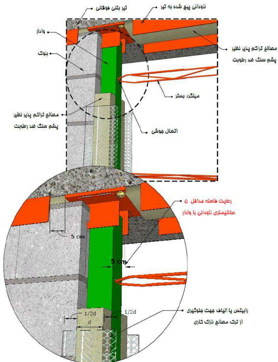
شکل پ ۴-۴-۴-۱-۶ اجرای عایق پشم سنگ و مش الیاف یا رابطیس بر روی وادار
