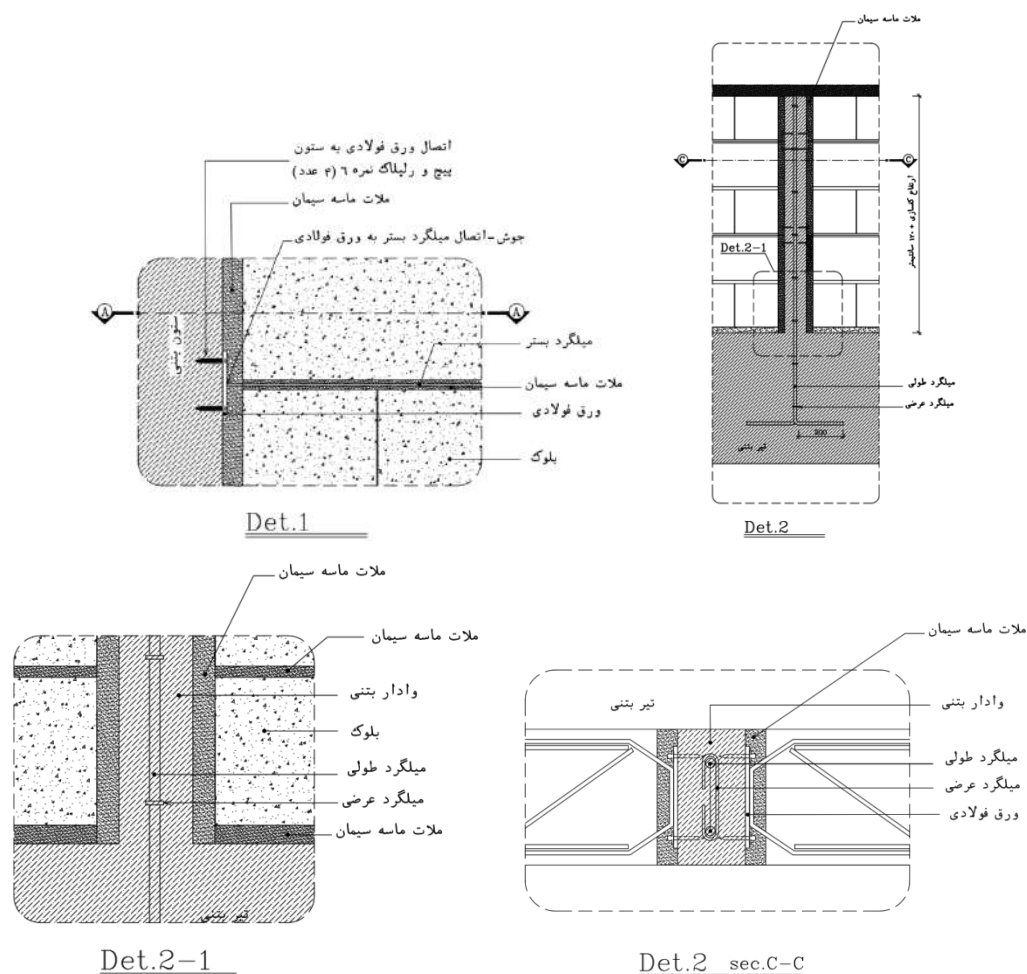
شکل پ ۳۷-۶- جزئیات اجرایی اتصال جان پناه با وادار بتنی
