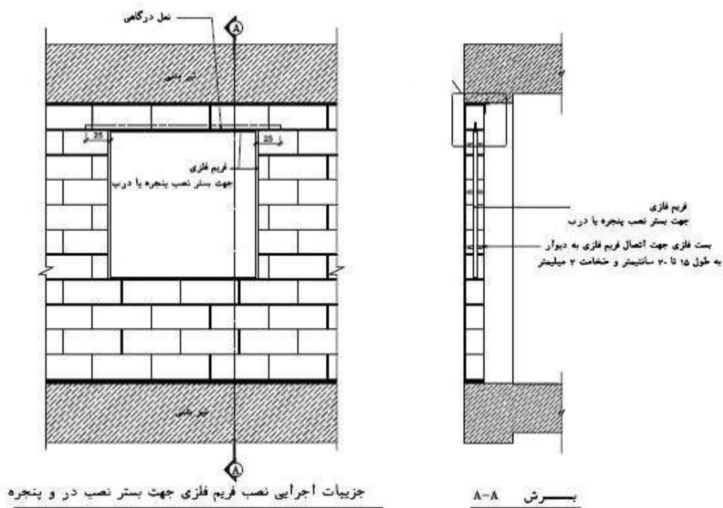
شکل پ ۶-۱۵- نحوه اجرای فریم و نعل درگاه در اطراف بازشو
