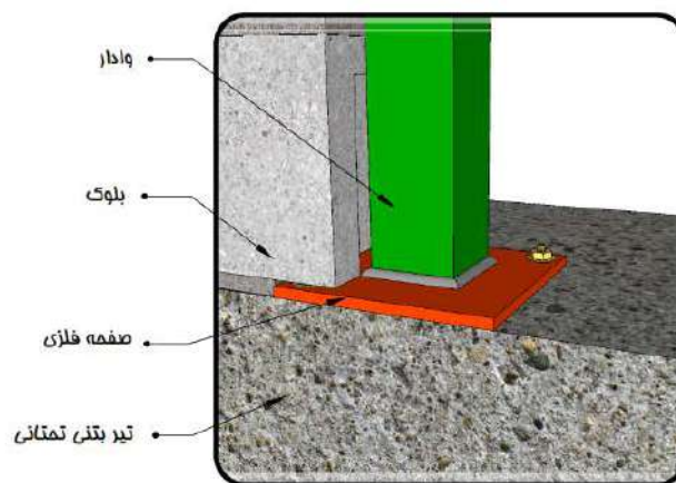
مزییات اتصال وادار میانی روی تیر تمثالی
